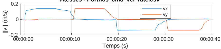
Vitesse - Porthos_cmd_vel_rate.csv
